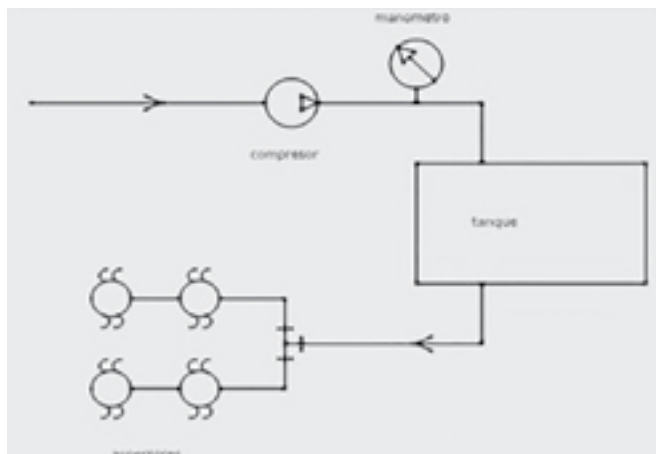
Fig. (1). Circuito hidráulico de distribución de aspersores (rociadores).
