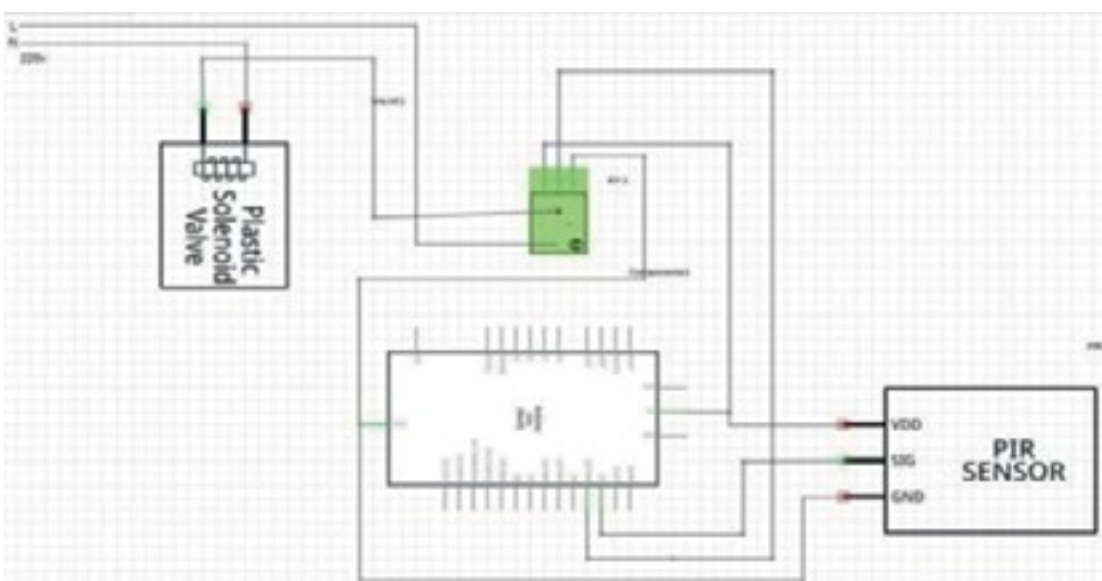
Circuito eléctrico esquemático
